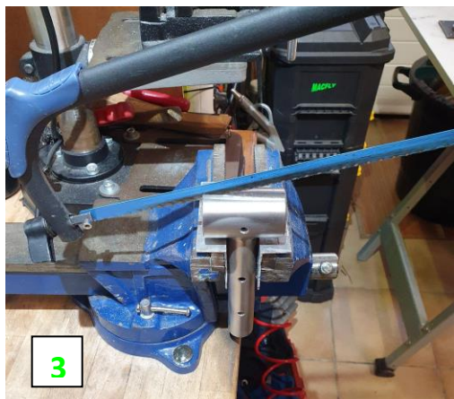
Découpe de la base du tube de support de siège avec une incision dans la longueur
